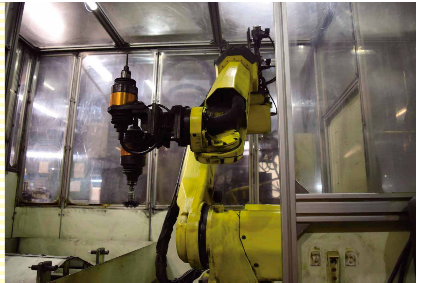
ロボットの活用でバリ取りの自動化を果たし、効率アップとコストダウンにつなげた
