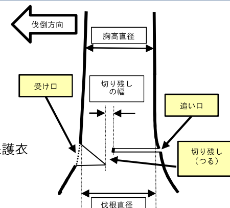
（図2）受け口、追い口等の関係図
